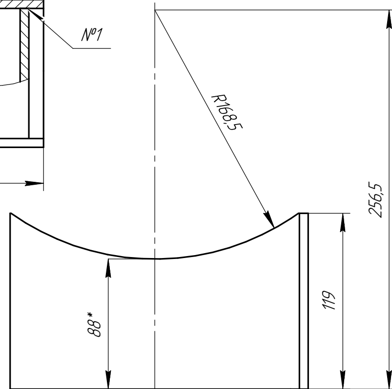
Дет. поз. 2
