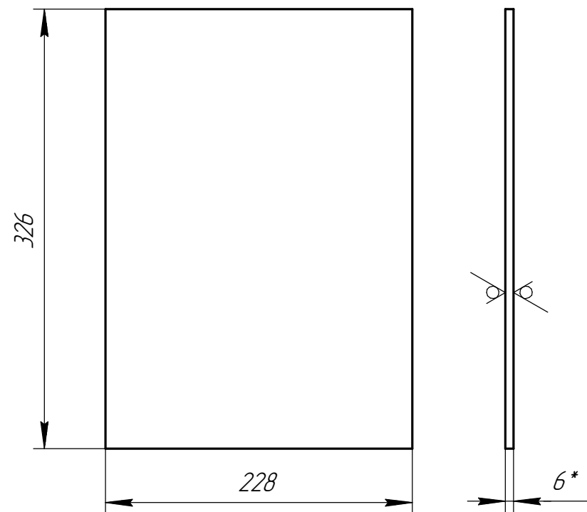
Дет. поз. 1 (1:4)
